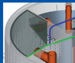
Abdeckung Wirbelschwebbettkammer mit Wartungsöffnung. Verhindert ein Abtreiben der Aufwuchskörper bei einem eventuellen Rückstau.
