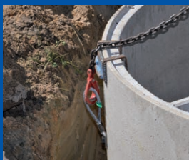
Seilschlaufen zum einfachen sicheren Versetzen der Betonbehälter. Mindestkettenlänge \geq 2,5 m.
