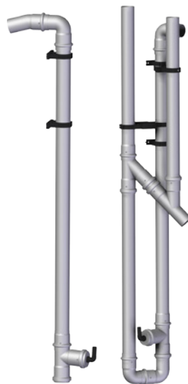
Rohrsystem STABI KOM
